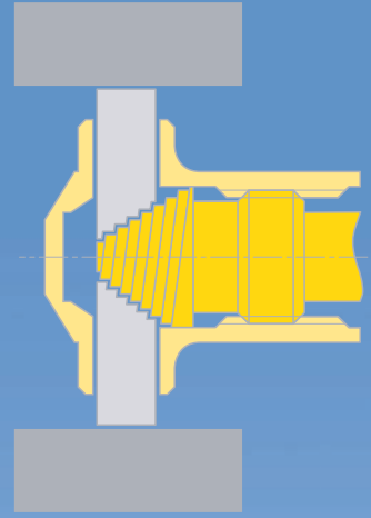
Mentes kúp kialakítás az Abbe elvnek megfelelően
