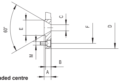
Centering insert Wkładka centrująca
