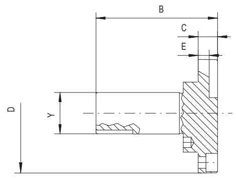
Centering insert Wkładka centrująca
